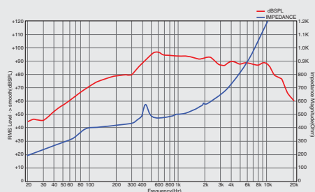
► CS-610F
