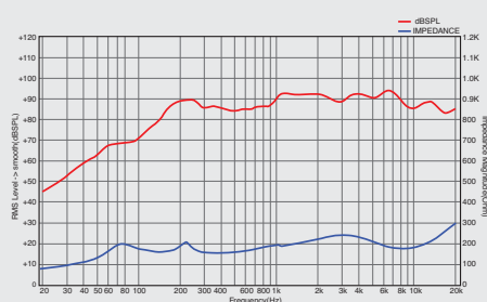
► CS-630FH
