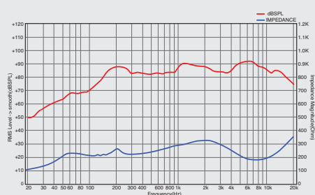
► CS-620FH
